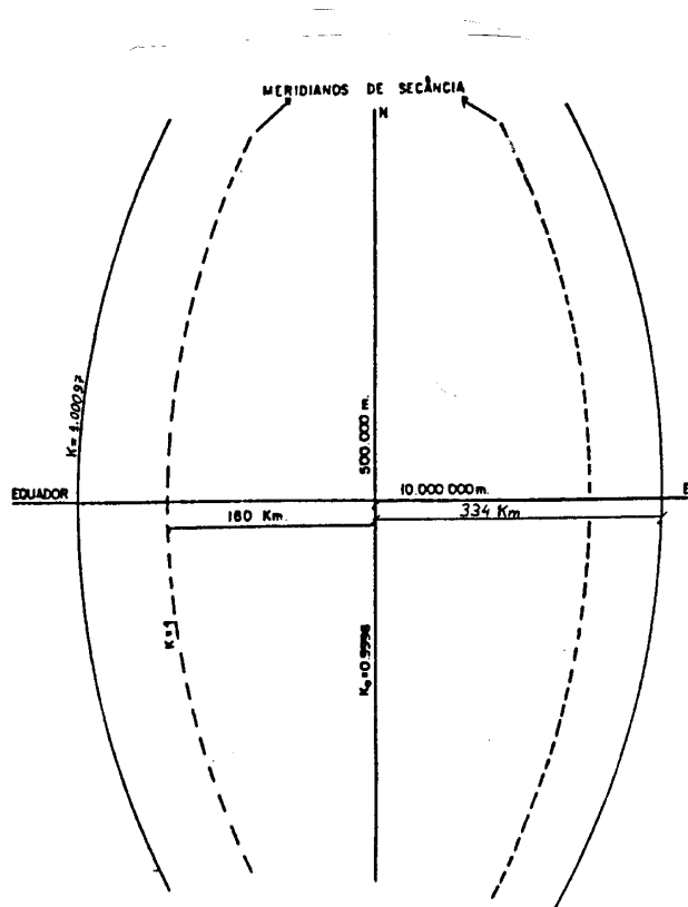
fig.2.12 - Fuso UTM com cilindro secante.
